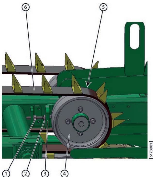
Fig. 83: Régler la tension des courroies
