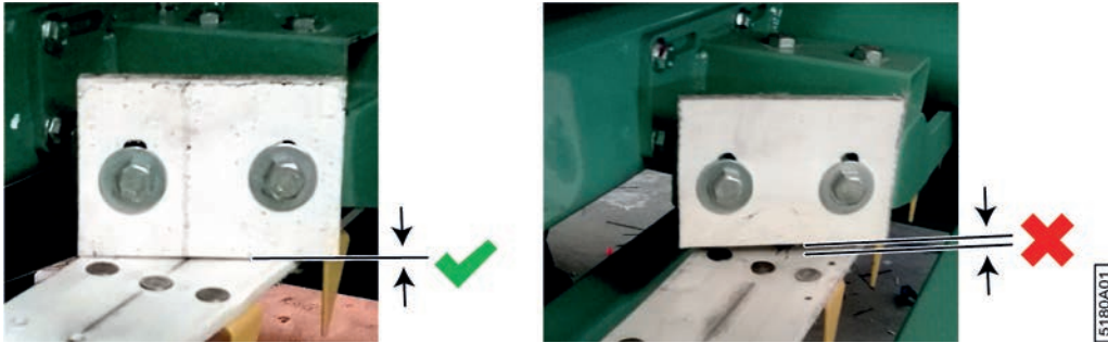
Fig. 97: Positionnement correct et incorrect du racleur
