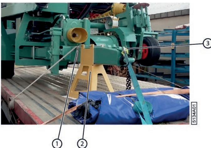
Fig. 44: Fixer la machine sur le camion (avant)
