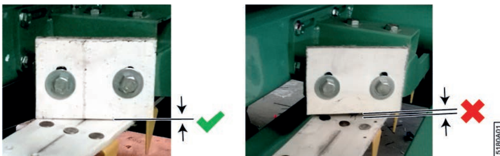
Fig. 123: Positionnement correct et incorrect du racleur
