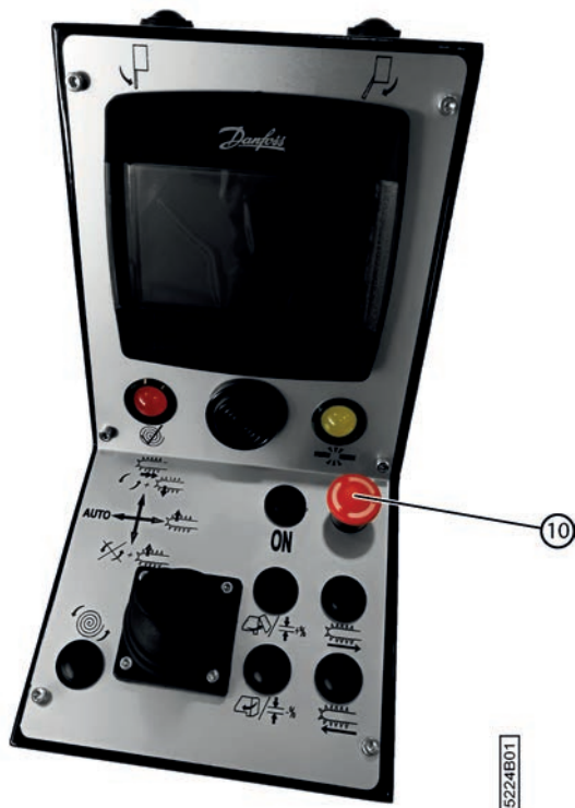
Fig. 95: Arrêter la machine
