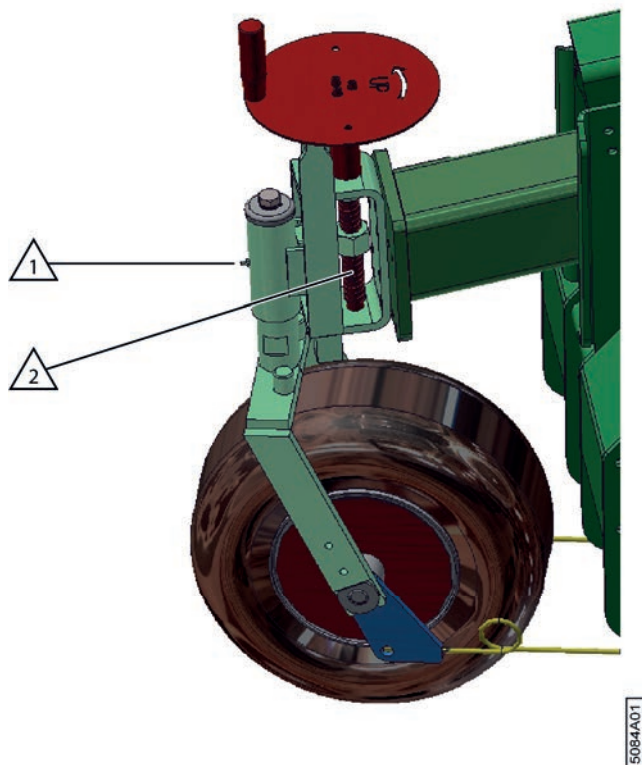
Fig. 113: Lubrifier la roue de jauge
