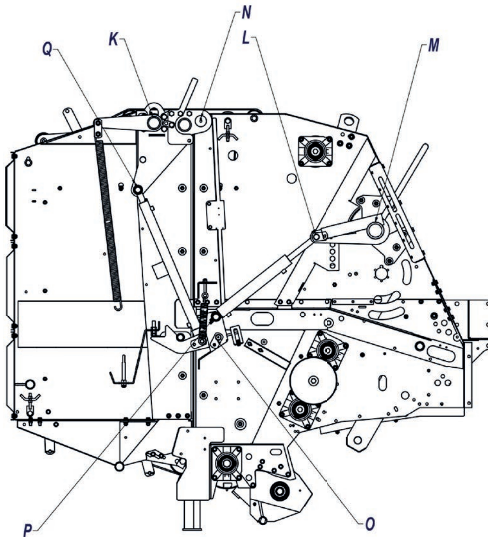
Fig. 115: Aperçu des points de graissage du côté droit de la cage
