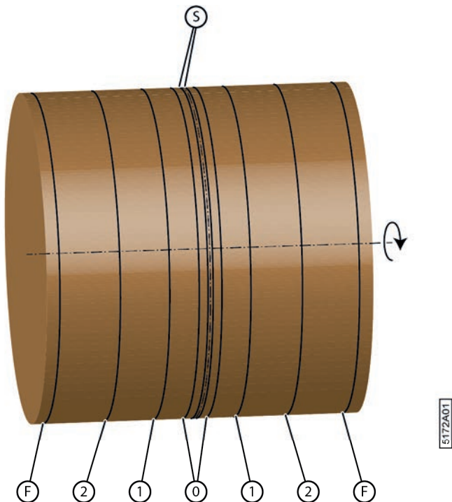
Fig. 76: Positions de la ficelle lors du liage
