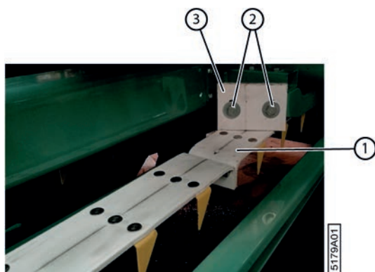
Fig. 85: Régler le racleur
