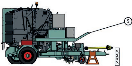
Fig. 140: Support de maintien
