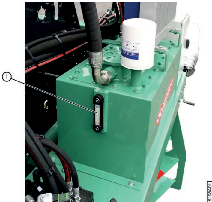
Fig. 106: Niveau huile hydraulique
