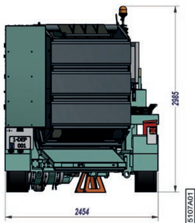
Fig. 5: Dimensions (largeur)
