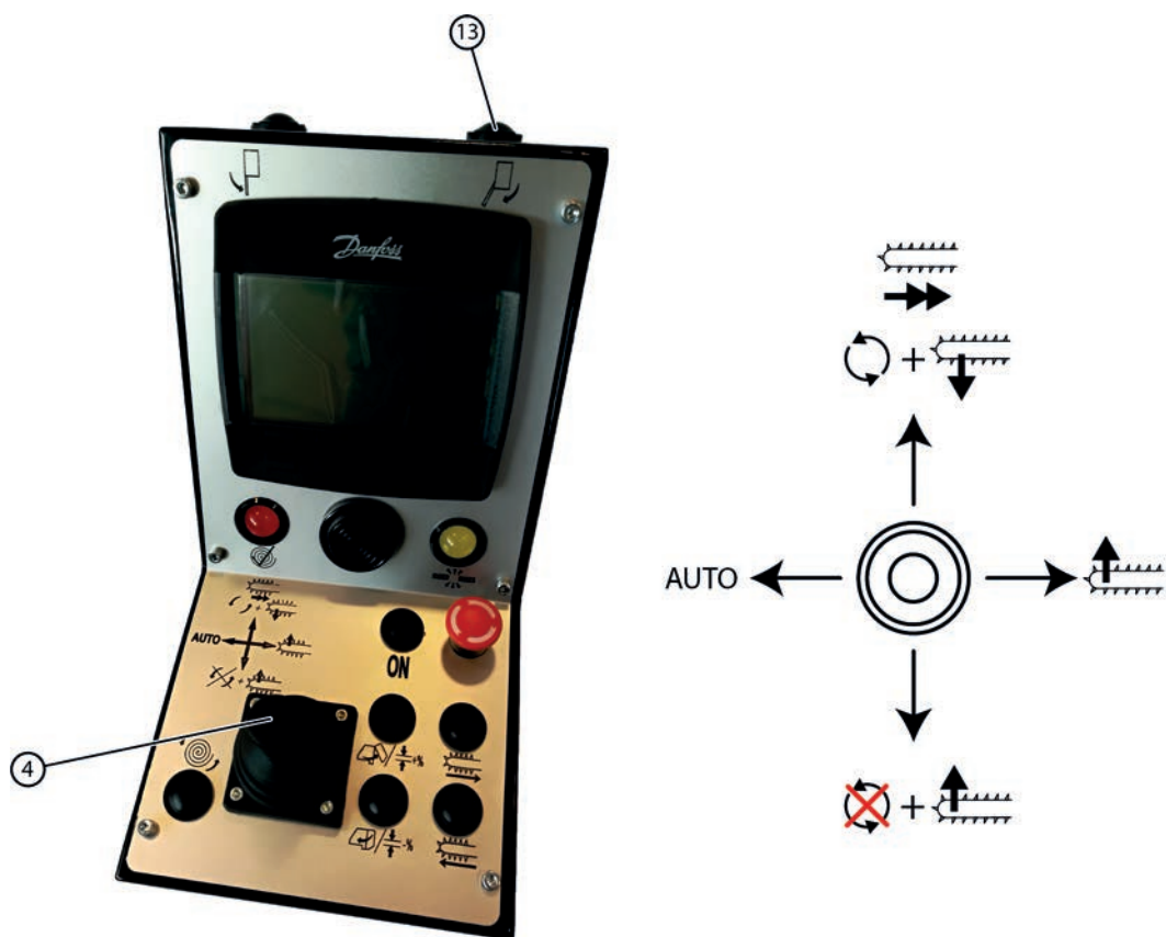
Fig. 66: Arracher le lin en l'enrouler (mode enroulement)
