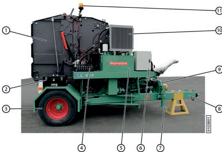
Fig. 6: Vue de côté à droite
