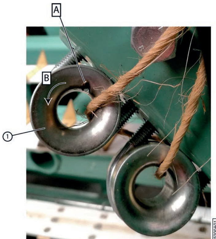
Fig. 111: Usure d'un guide ficelle
