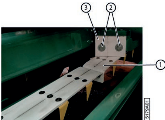
Fig. 98: Positionnement correct du racleur
