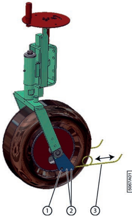
Fig. 82: Réglages possibles de la roue de jauge
