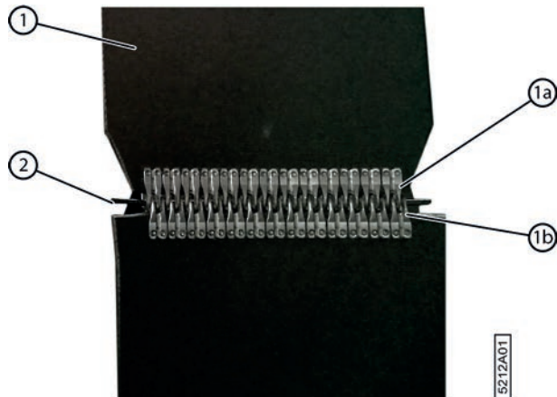
Fig. 129: Remplacer les courroies de cage
