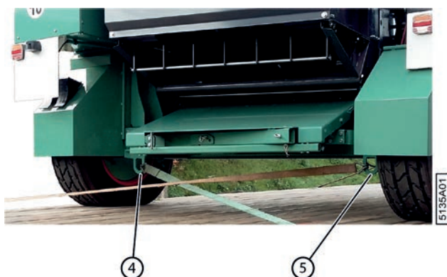
Fig. 45: Fixer la machine sur le camion (arrière)
