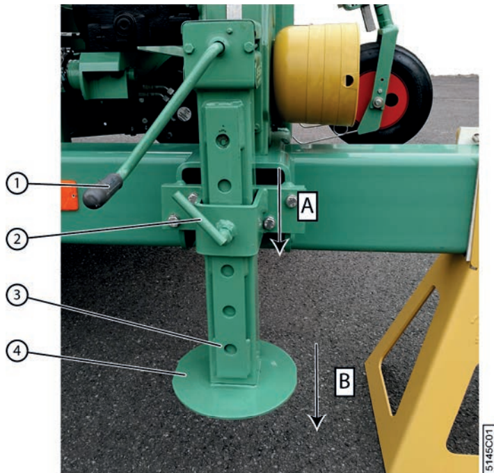
Fig. 141: Déployer béquille mécanique
