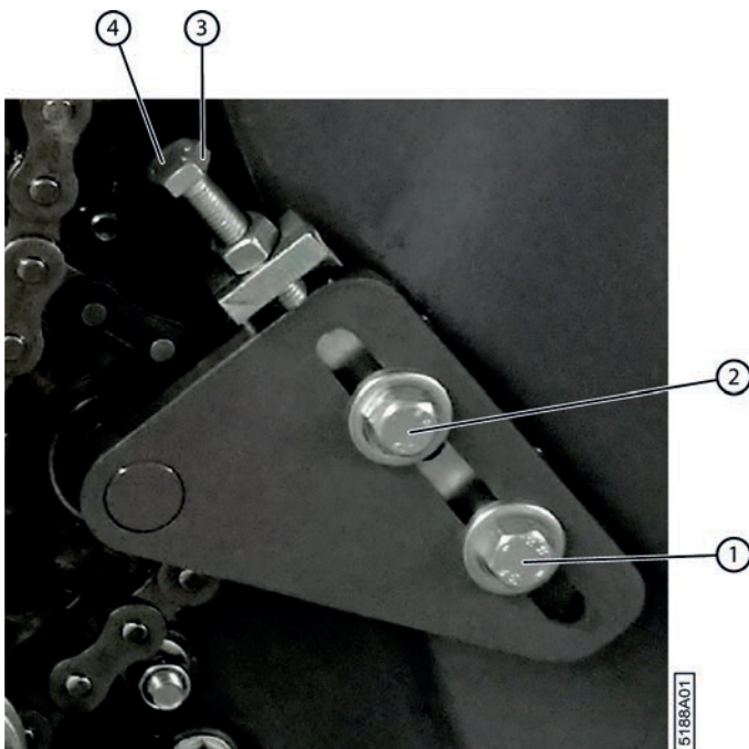
Fig. 93: Régler le tendeur de chaîne manuel
