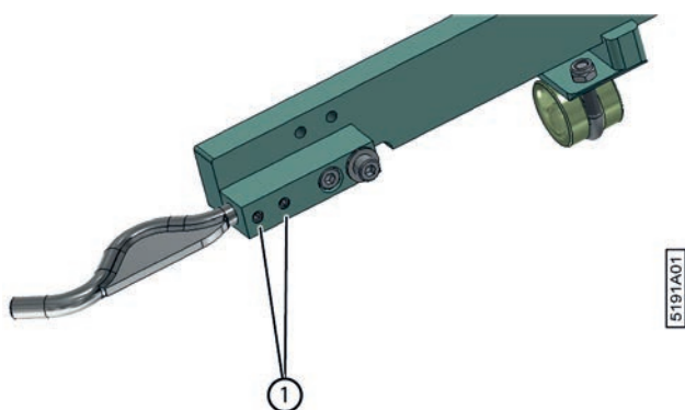
Fig. 133: Remplacer les doigts du système de liage par ficelle
