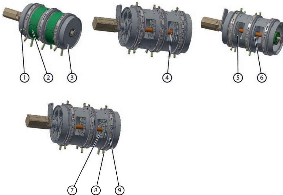
Fig. 127: Replacer la dent du tambour de pick-up
