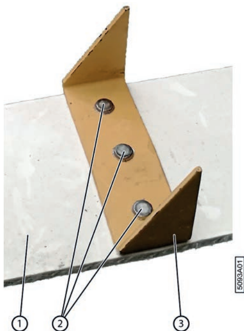
Fig. 134: Remplacer un picot
