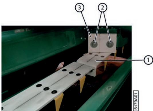
Fig. 122: Démontant le racleur
