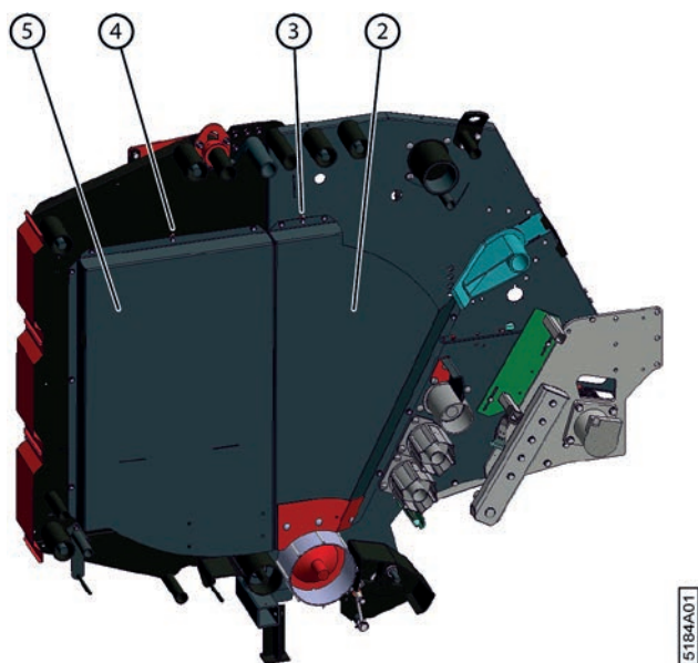
Fig. 89: Monter une tôle côté tête
