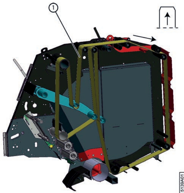
Fig. 126: Remplacer les courroies de cage cassées
