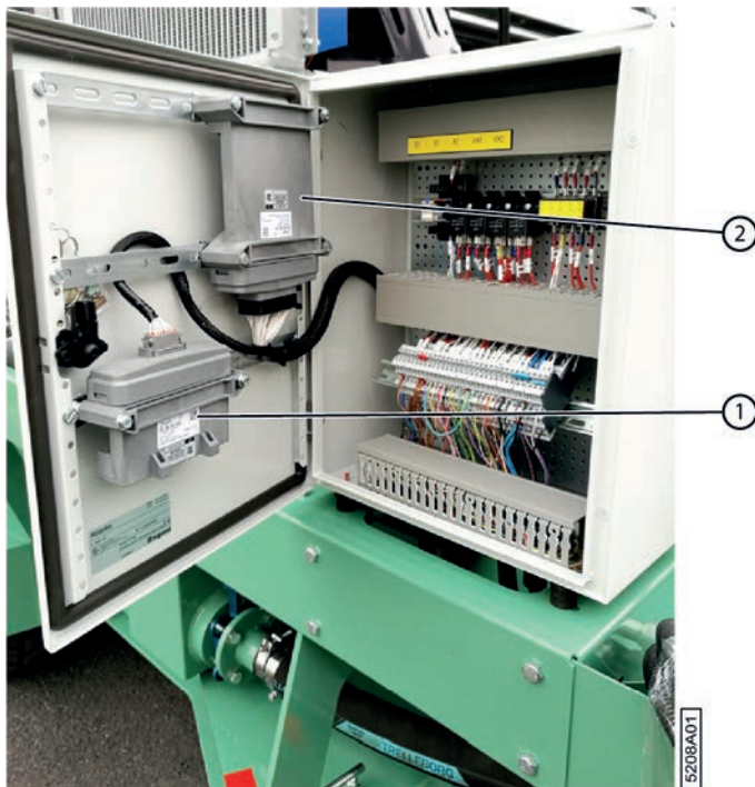
Fig. 121: Emplacement des contrôleurs
