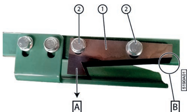
Fig. 131: Remplacer un couteau
