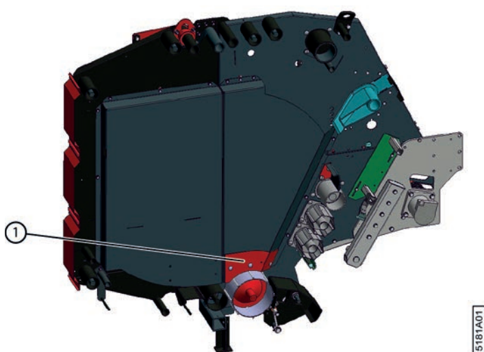
Fig. 130: Remplacer la tôle d'usure
