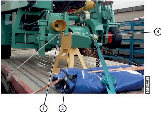
Fig. 41: Fixer la machine sur le camion (avant)
