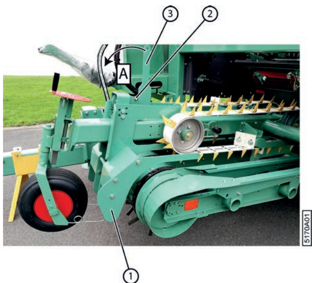
Fig. 70: Ouvrir le contre pick-up
