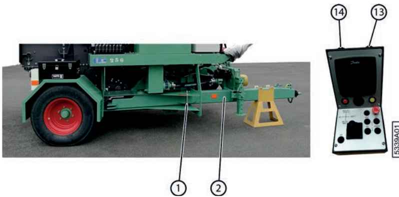
Fig. 61: Commande du timon
