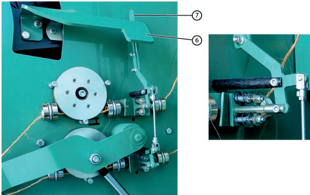
Fig. 138: Le levier du système de tension ficelle
