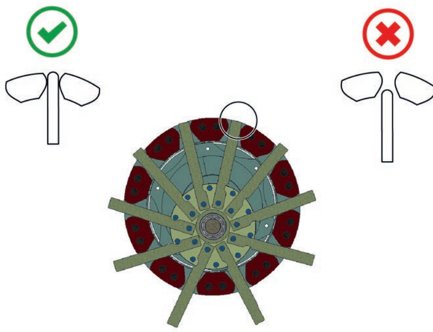
Fig. 102: Les dents du pick-up
