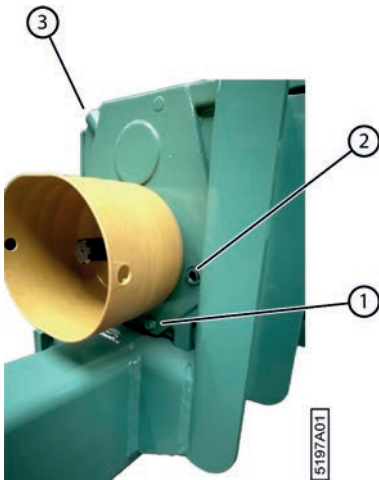
Fig. 104: Vérifier le niveau d'huile dans le réducteur
