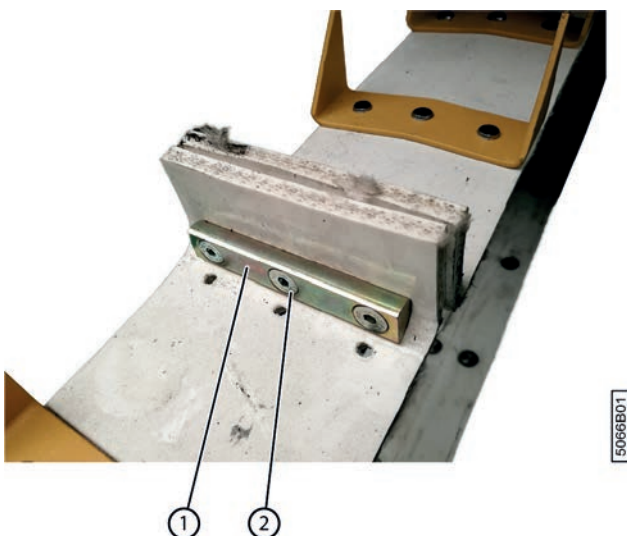
Fig. 124: Remplacer une courroie de transport
