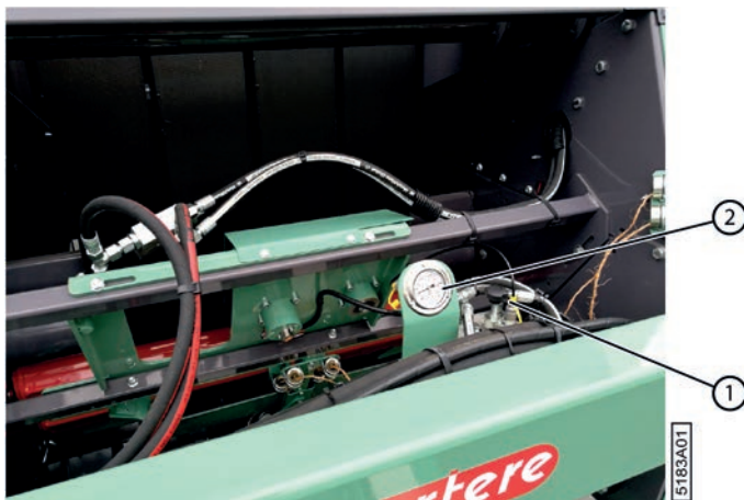
Fig. 88: Régler la pression de serrage dans la cage
