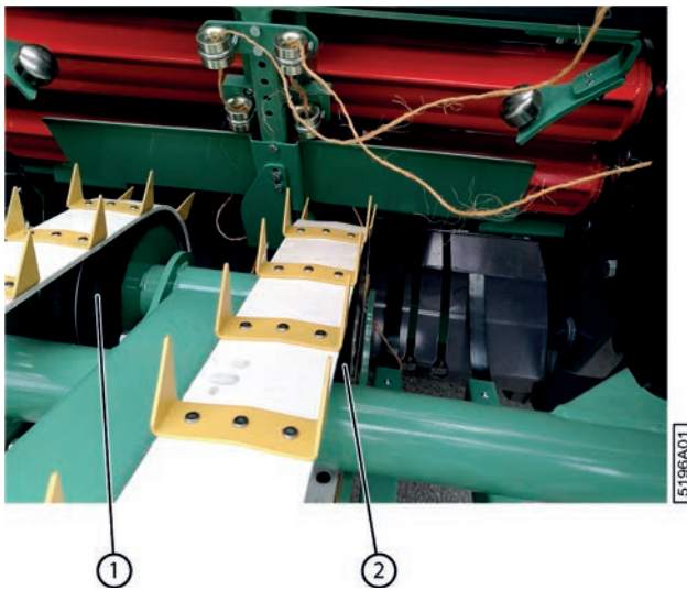
Fig. 103: Contrôler les rouleaux d'entraînement
