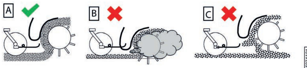
Fig. 79: Réglages possibles de la hauteur du pick-up
