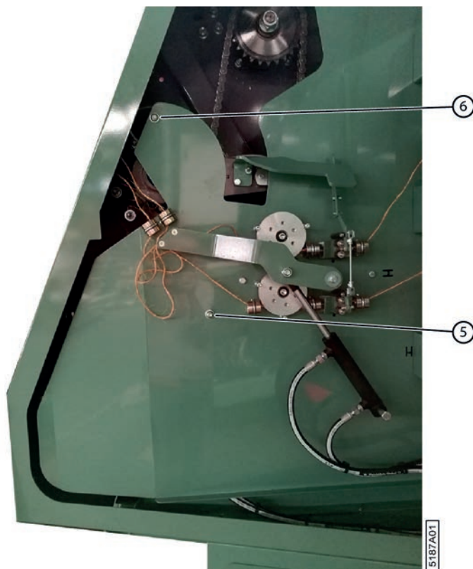
Fig. 92: Protection du compartiment à ficelle
