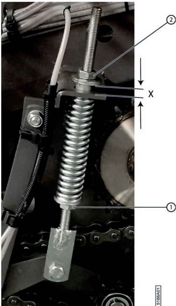
Fig. 91: Régler le tendeur de chaîne automatique
