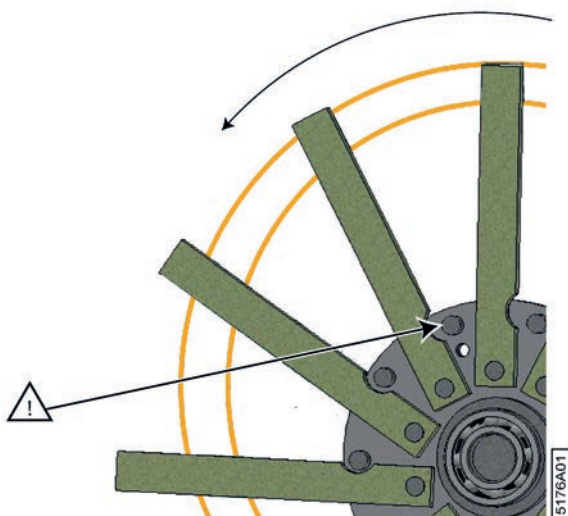
Fig. 128: Placement d'une nouvelle dent
