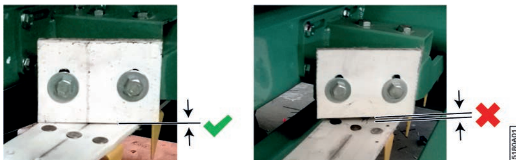
Fig. 86: Positionnement correct et incorrect du racleur
