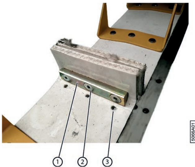
Fig. 84: Raccourcir les courroies de transport
