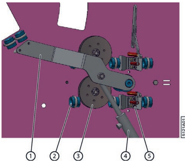
Fig. 27: Système de tension ficelle
