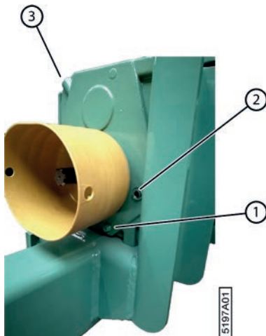
Fig. 105: Remplacer l'huile du réducteur
