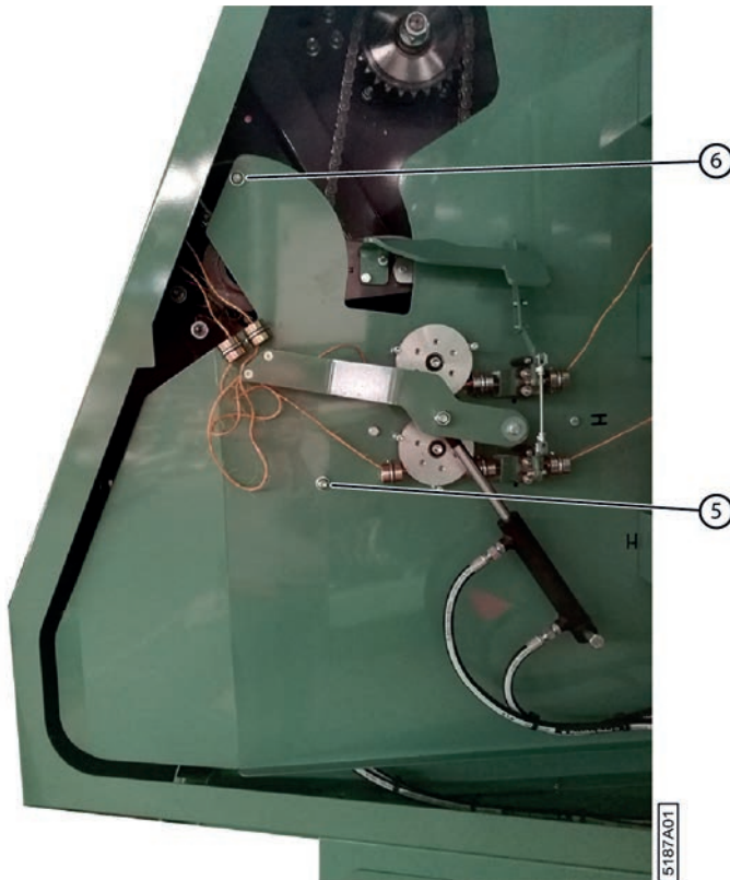
Fig. 108: Protection du compartiment à ficelle
