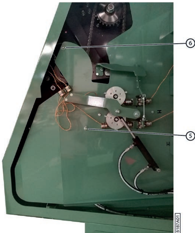
Fig. 94: Protection du compartiment à ficelle
