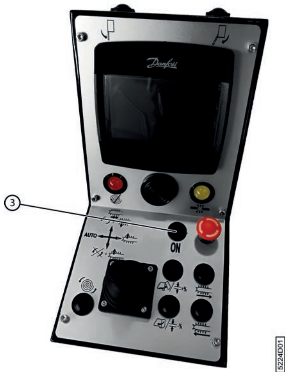
Fig. 62: Démarrer la machine
