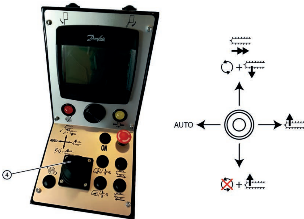
Fig. 65: Lever/abaissier le pick-up avec le joystick
