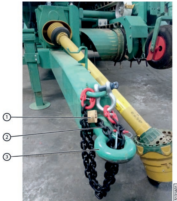
Fig. 36: Sécurisation contre le vol
