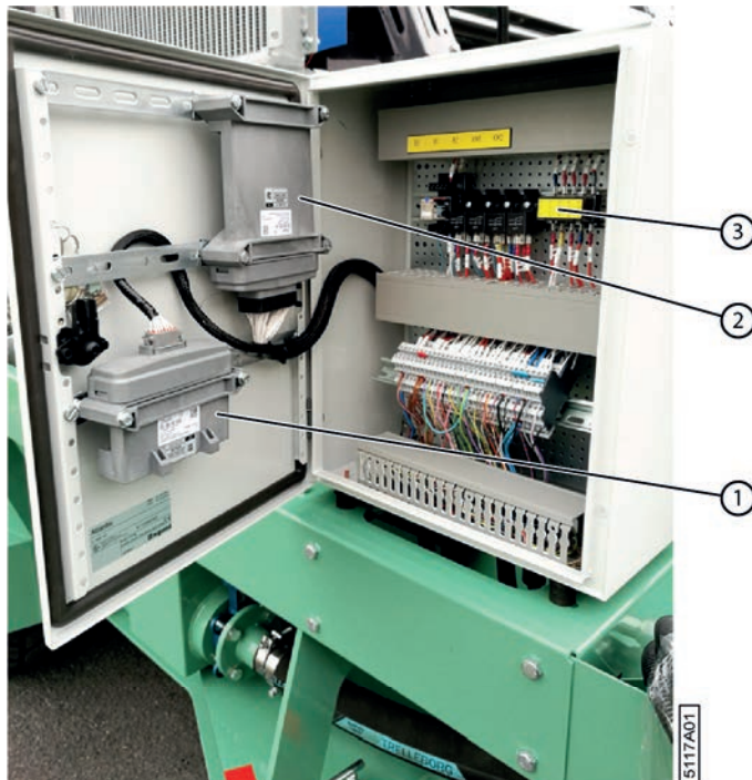
Fig. 17: Armoire électrique
