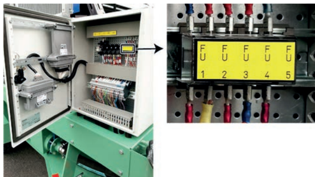
Fig. 135: Remplacer un fusible dans l'armoire électrique
