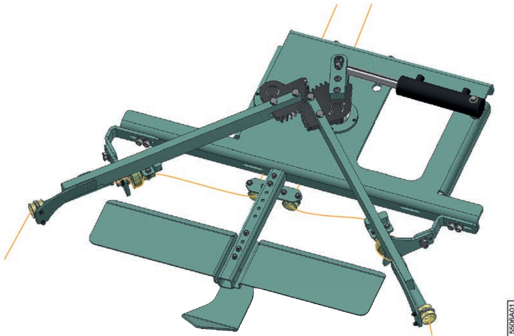
Fig. 26: Le système de liage par ficelle avec les ficelles en position ouverte (vue de dessous)
