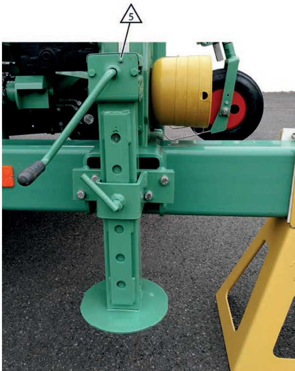
Fig. 118: Lubrifier la béquille mécanique
