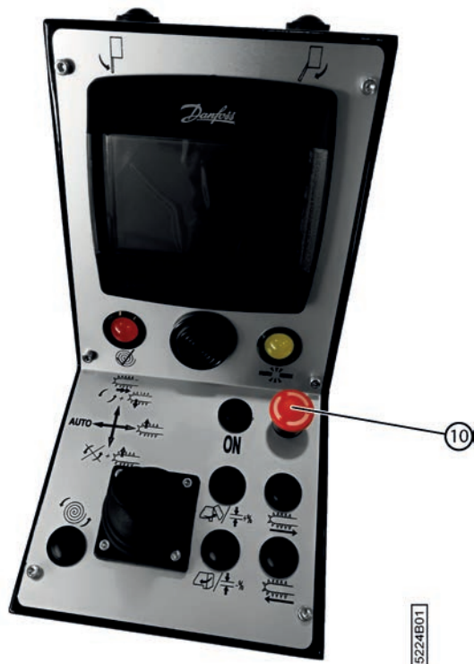
Fig. 63: Arrêter la machine
