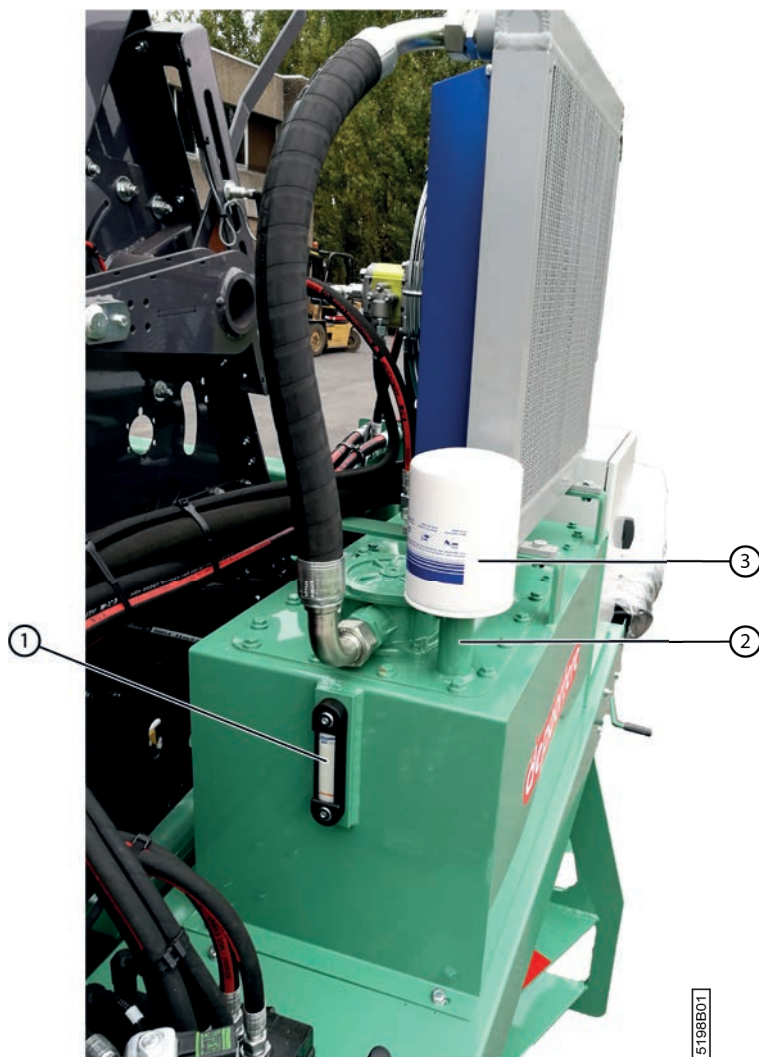
Fig. 107: Remplacer l'huile hydraulique
