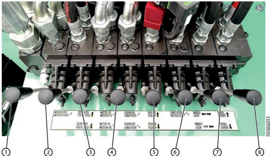
Fig. 60: Bloc de soupapes
