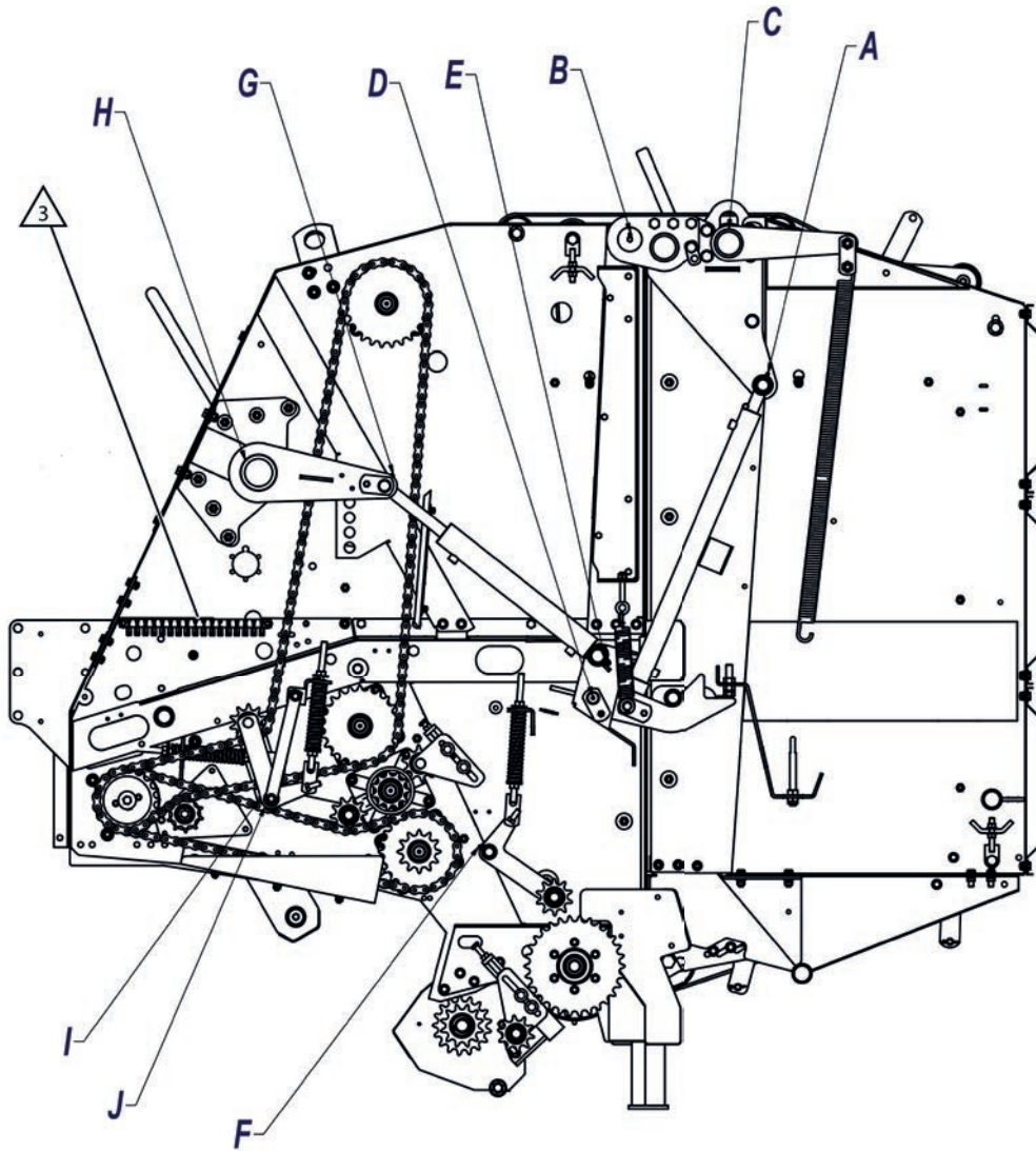
Fig. 114: Aperçu des points de graissage du côté gauche de la cage
