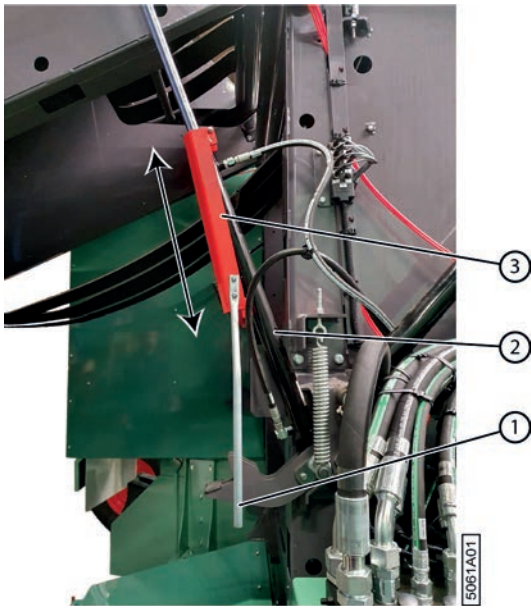
Fig. 96: Verrouiller la cage
