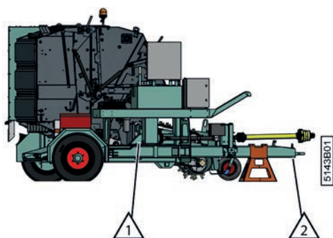
Fig. 116: Lubrifier le timon
