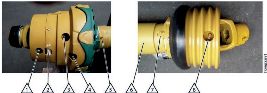
Fig. 119: Lubrifier le cardan
