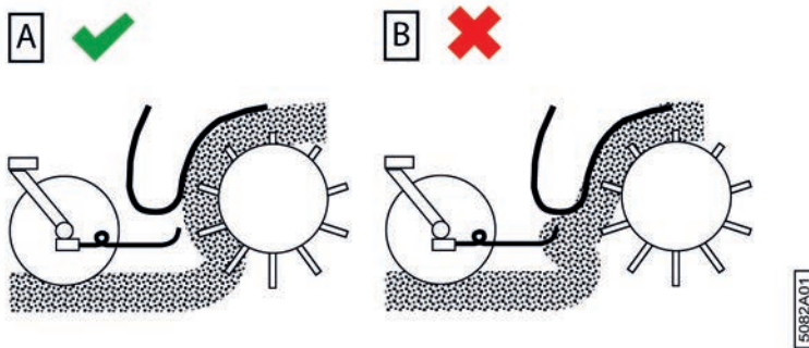
Fig. 81: Réglages possibles de la roue de jauge
