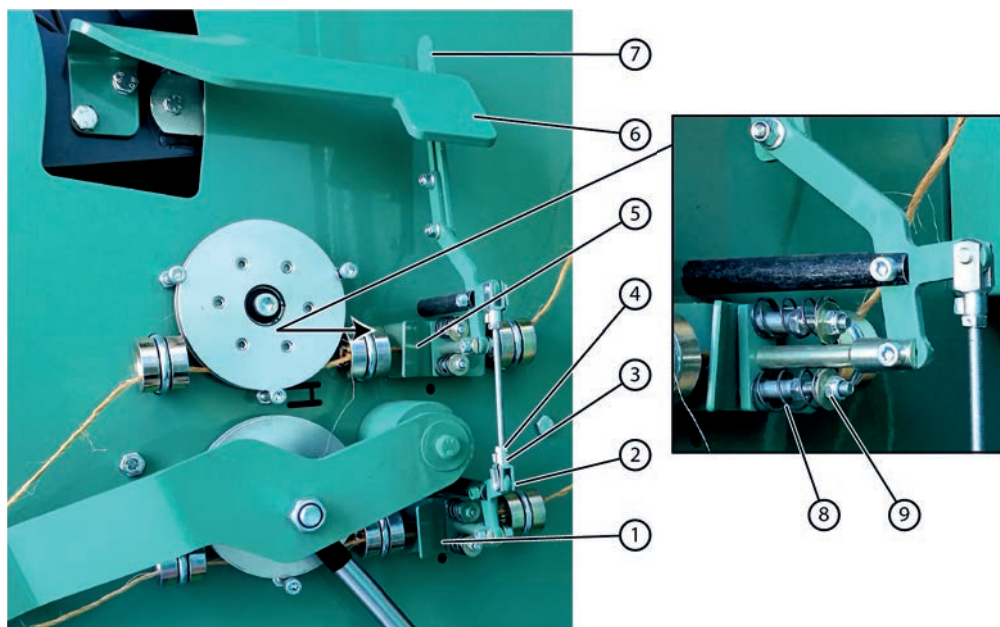
Fig. 87: Régler les tendeurs ficelles
