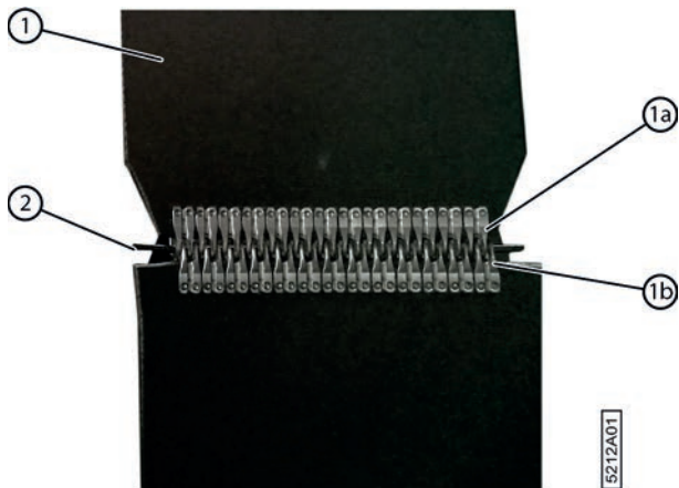
Fig. 125: Remplacer les courroies de cage
