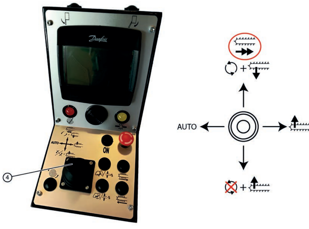
Fig. 75: Fonction Boost
