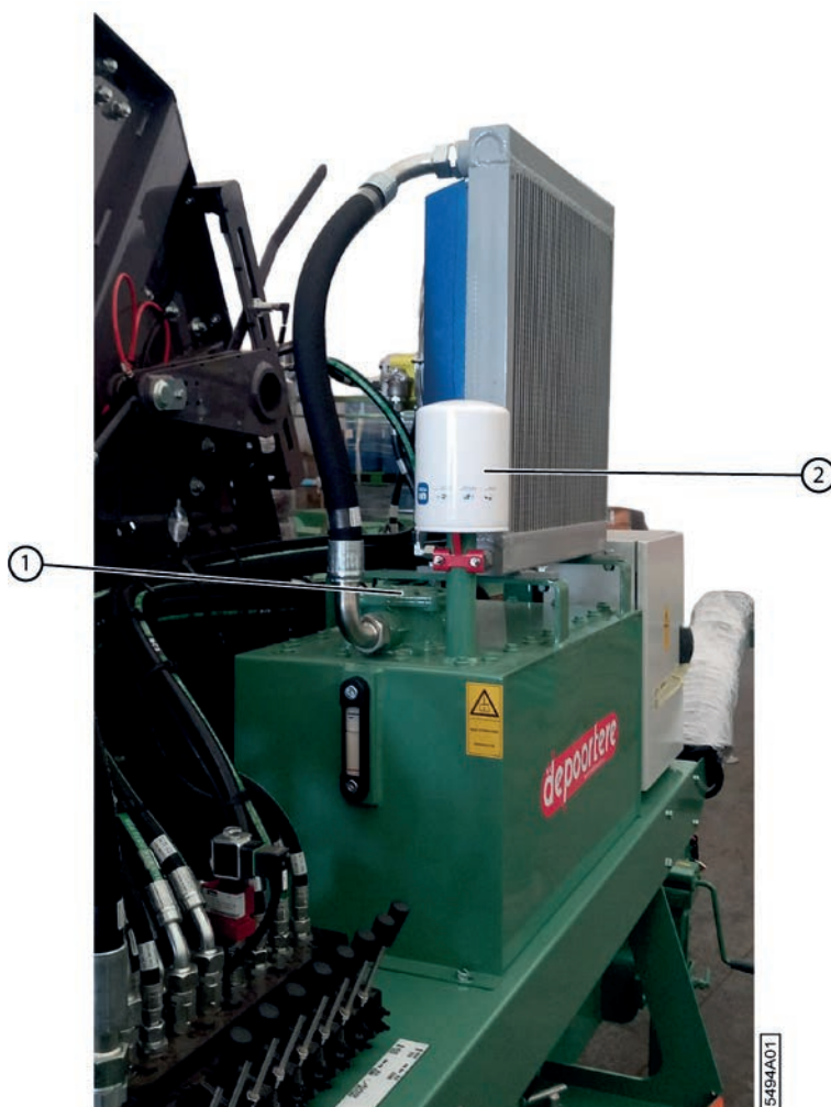
Fig. 144: Filtre de retour et reniflard
