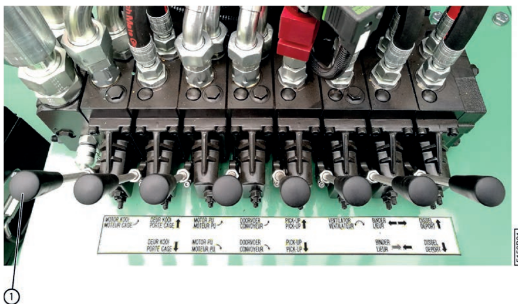
Fig. 112: Bloc de soupapes
